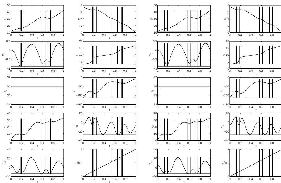
FIG. 4.15 – Transfert 2D à masse constante, 24 Newtons, couplage avec l'homotopie. Les graphes de gauche et de droite correspondent à la même solution, mais à gauche, la grille est celle sur laquelle la résolution a été effectuée, à droite celle que l'on peut calculer à partir de la solution elle-même, et qui sert pour la poussée suivante.
