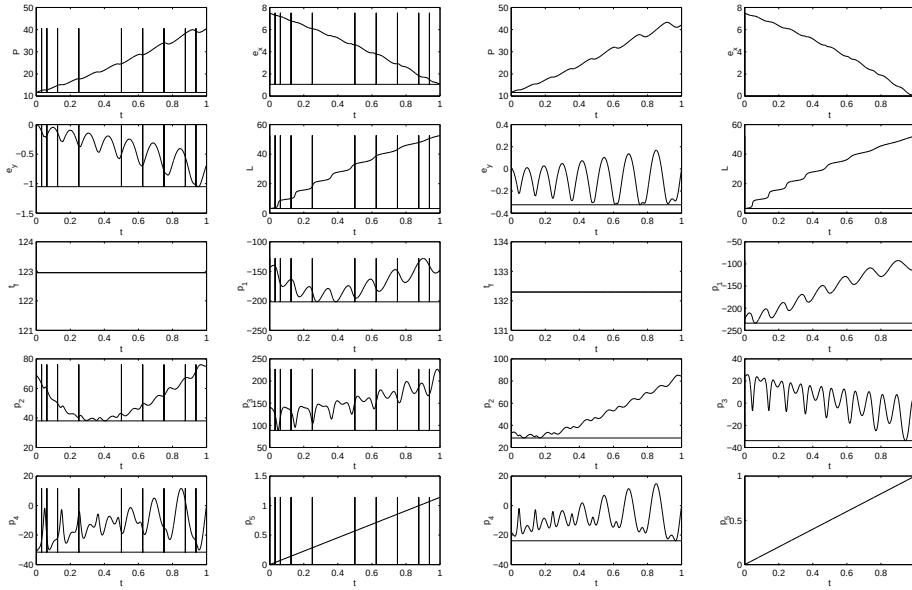
FIG. 4.14 – Transfert 2D à masse constante, 7 Newtons, couplage avec l’itération non-linéaire. Le graphe de gauche donne l’allure de l’approximation obtenue par tir simple avec une tolérance \text{tol} = 0.1 . On calcule, à partir de cette approximation, une grille de N = 10 instants de tir—grille que l’on a superposée au graphe—que l’on utilise pour terminer la résolution en tir multiple. La solution finale est représentée par le graphe de droite.
