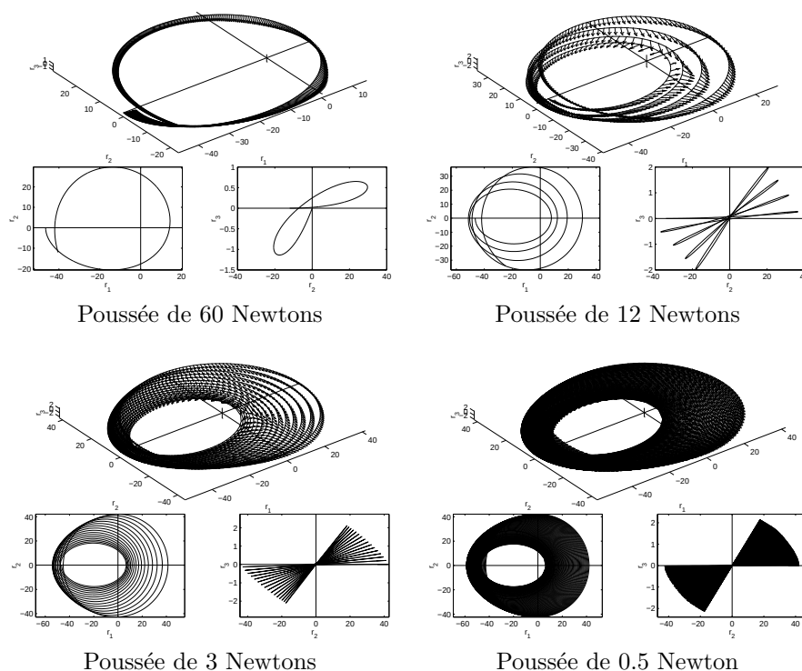
FIG. 5.7 – Transfert 3D à masse variable. Les trajectoires associées aux résultats de la figure 5.6 sont représentées en 3D (les flèches figurant l'action du contrôle), puis en projection sur les plans (r_1, r_2) et (r_2, r_3) . On voit en particulier comment, de tour en tour, on corrige l'excentricité dans le premier plan, et l'inclinaison dans le second.
