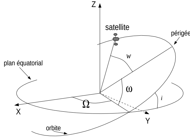
FIG. 1.1 – Éléments orbitaux.
